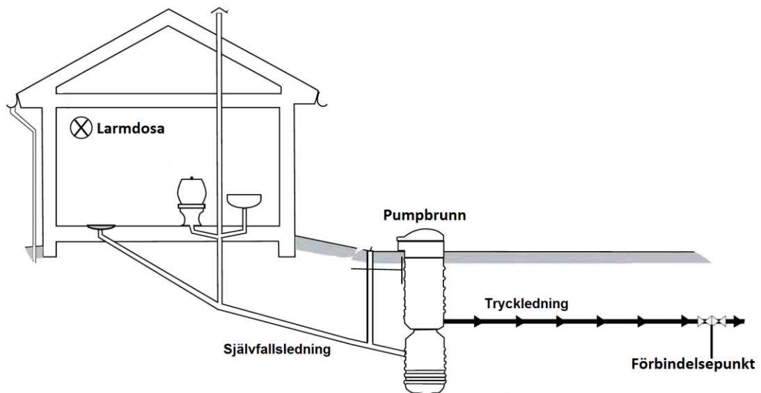
Avloppsinstallationen för ett normalt hushåll
